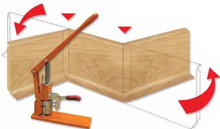
Stanzbare Verlegung mit der BOLTA Sockelleisten-Stanze Fast and easy installation, soft edges conform to surface irregularities
