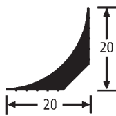
Artikel / Item 20 299 20 / 20 mm
