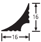
Artikel / Item 20 000 16 / 16 mm
